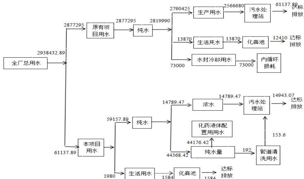
图 2-3 全厂水平衡图 (t/a)
