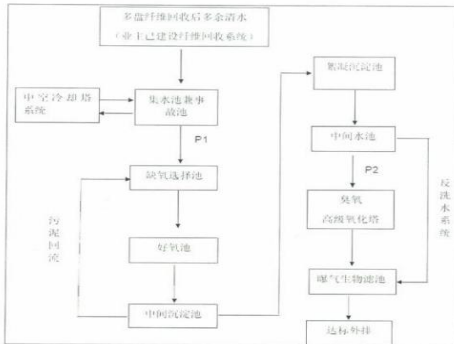
图4-4 废水处理工艺流程
