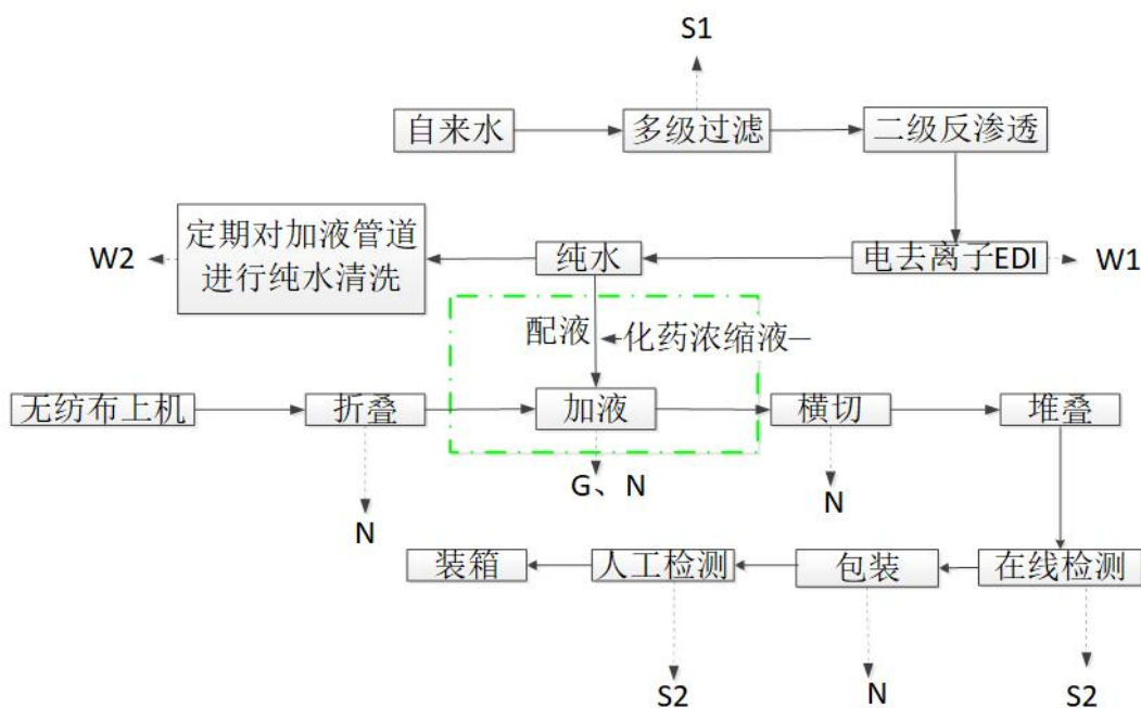
图2-4工艺流程及产排污节点图
