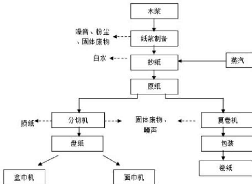
图 1 项目产污环节示意图
