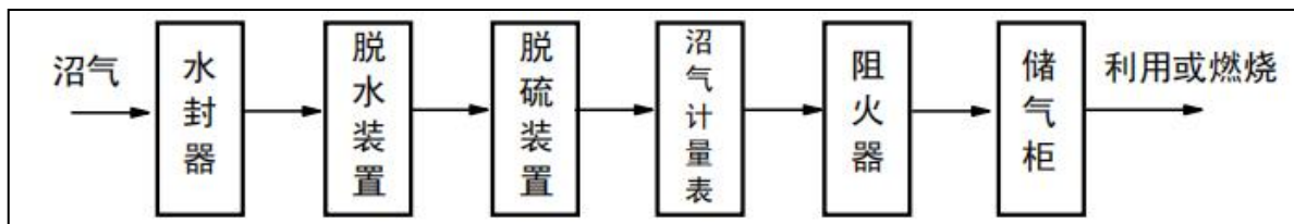
图 4-1 沼气利用方案
