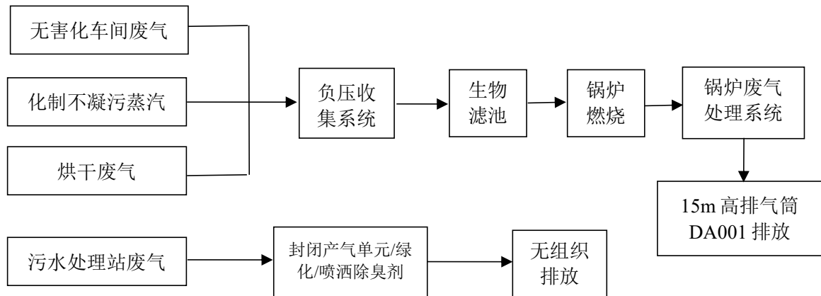
图 4-2 本项目恶臭废气处理路线示意图
