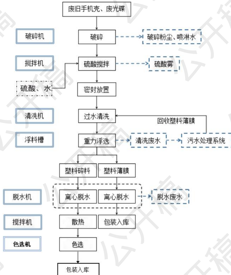
图 2-1 项目生产工艺流程图
