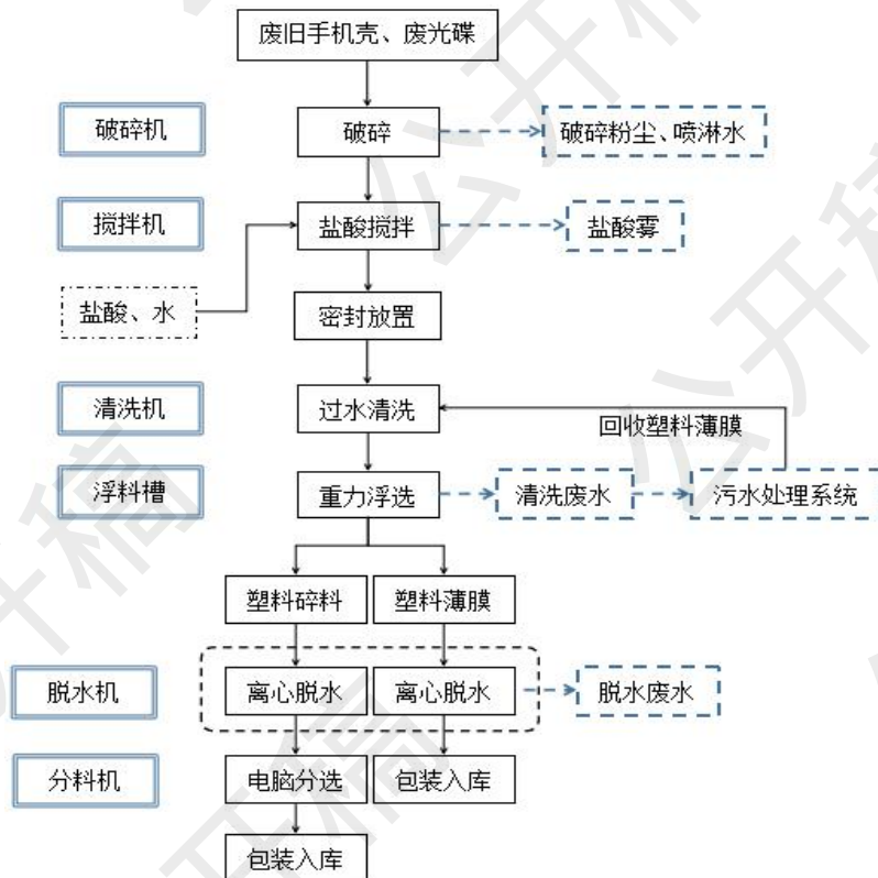
图 2-2 现有工程生产工艺流程图
