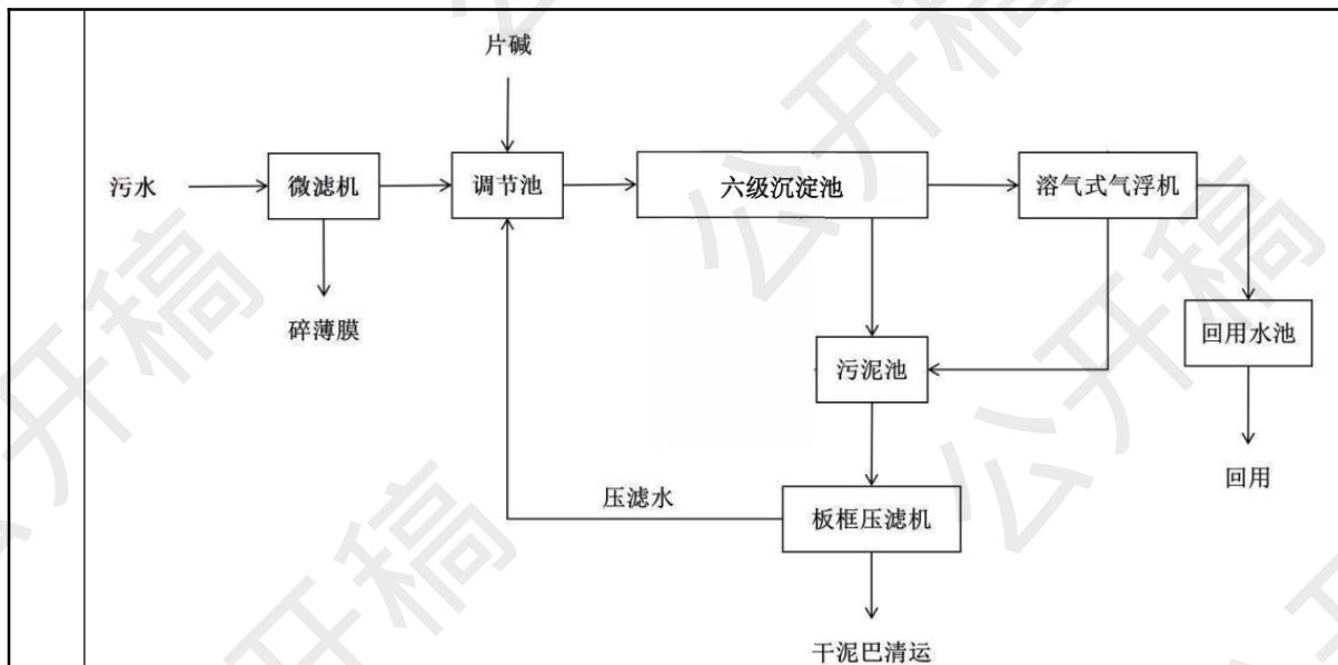
图 4-1 项目污水处理系统 (TW001) 工艺流程图
