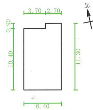
首层平面图 1:200
