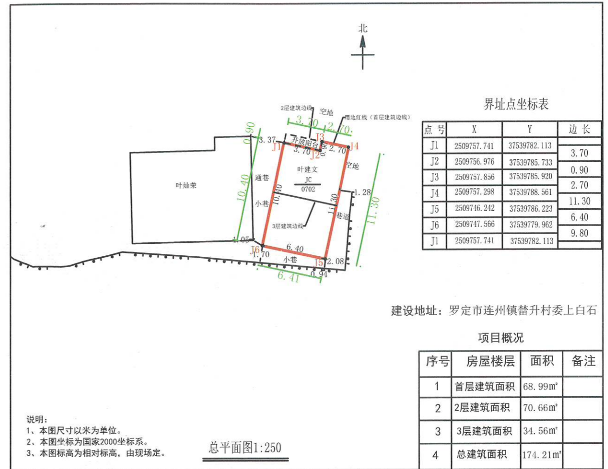
罗定市连州镇替升村委上白石叶建文建房平面图
