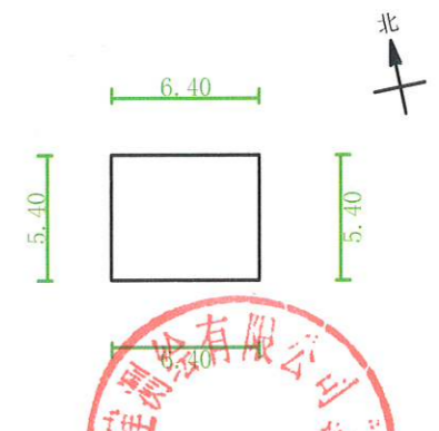
三层平面图 1:200
