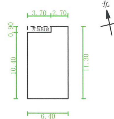
二层平面图 1:200
