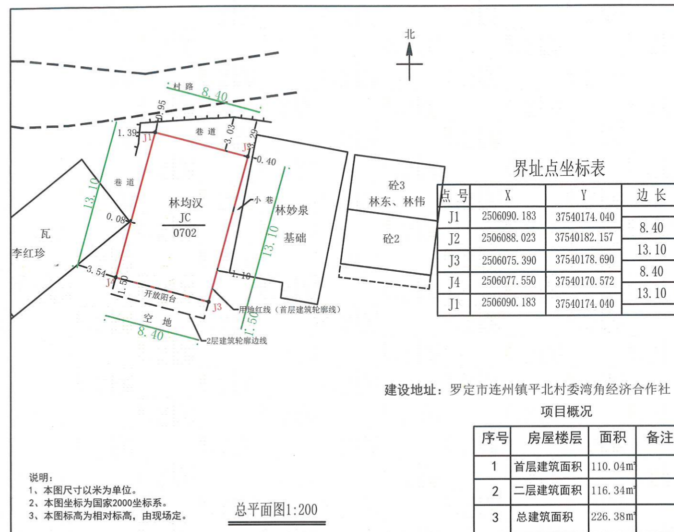
罗定市连州镇平北村委湾角经济合作社林均汉建房平面图
