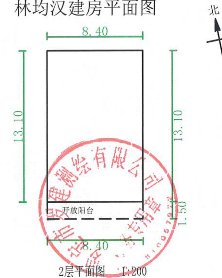
罗定市连州镇平北村委湾角经济合作社林均汉建房平面图
