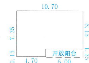
二至三层平面图 1:100 (每层层高: 3.20m) 注: 1、二至三层每层建筑面积: 75.50m 2
