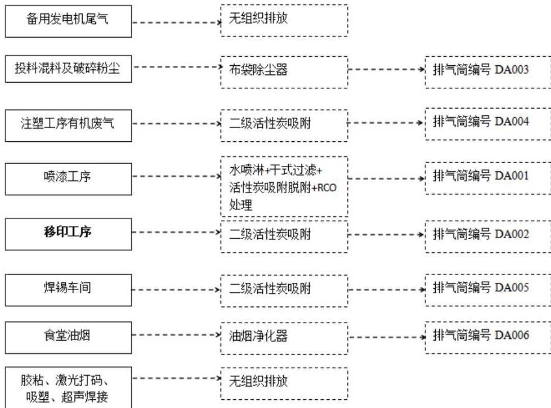
图 2-5 项目废气处理措施及排放方式
