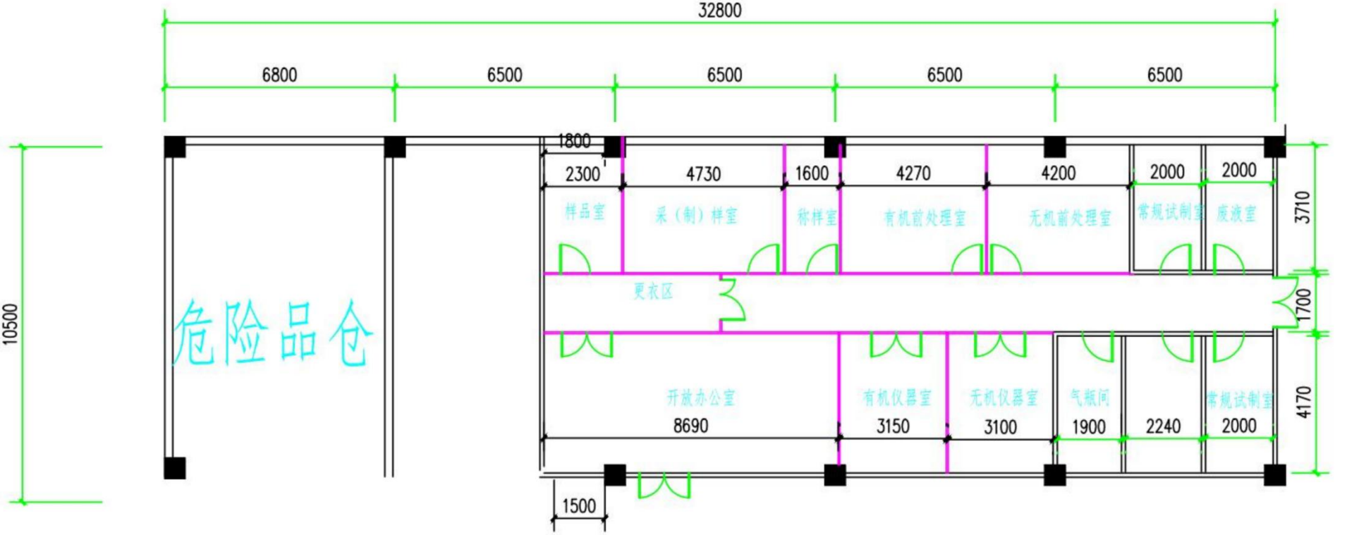
附图6 检测实验室平面布置图
