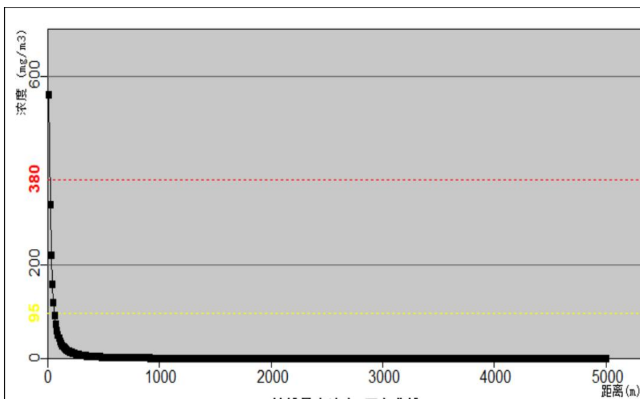
图 6.1-3 一氧化碳浓度随距离的变化曲线图
