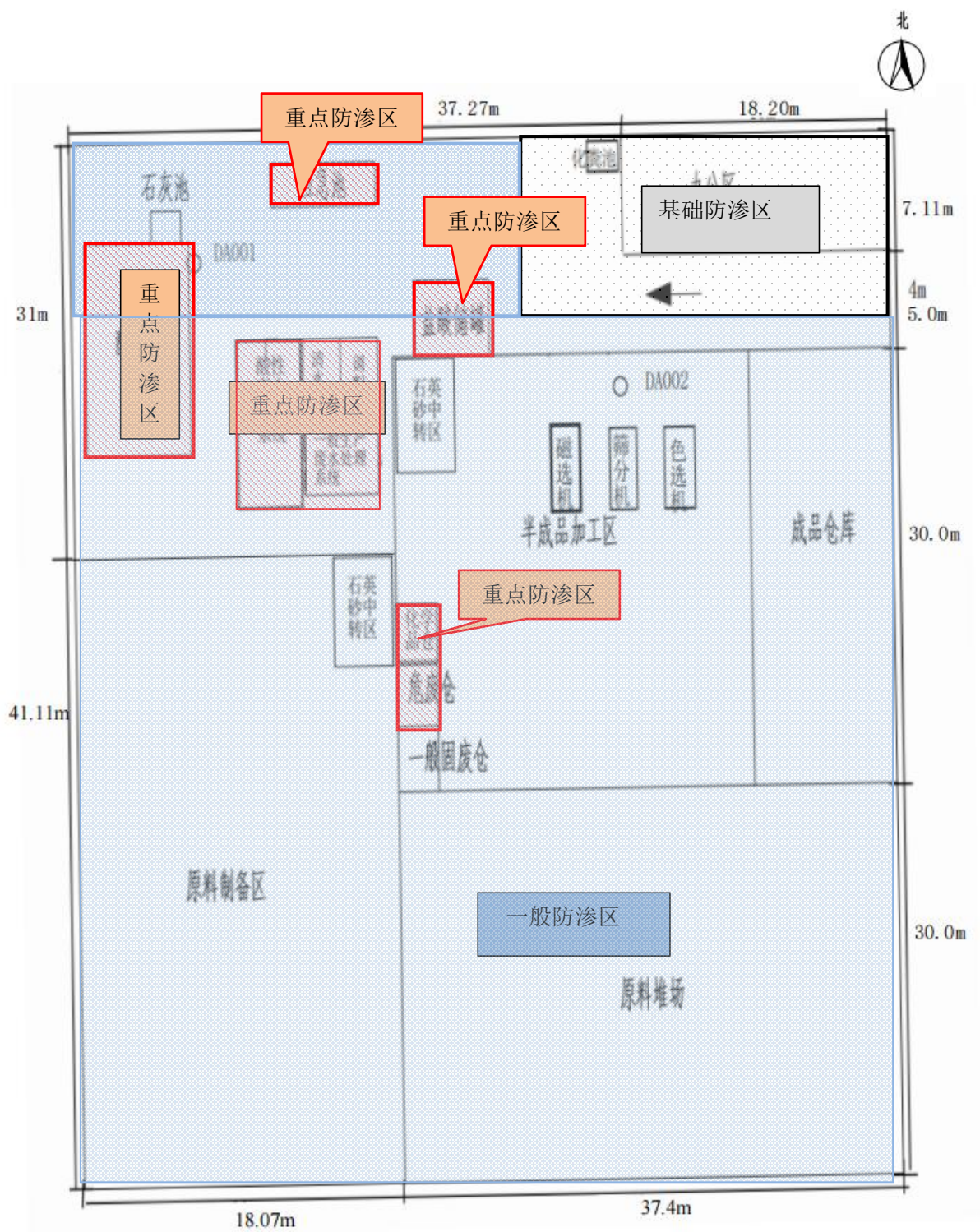
图 6.4-2 项目车间地下水防渗图
