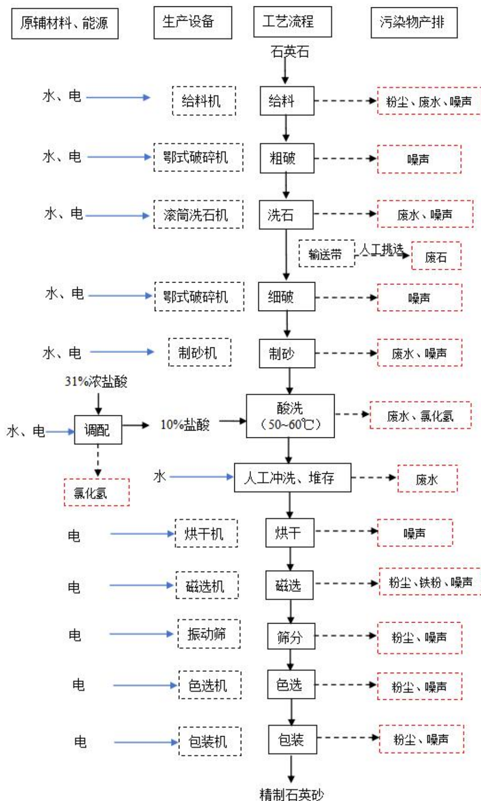
图2-3 精制石英砂工艺流程图
