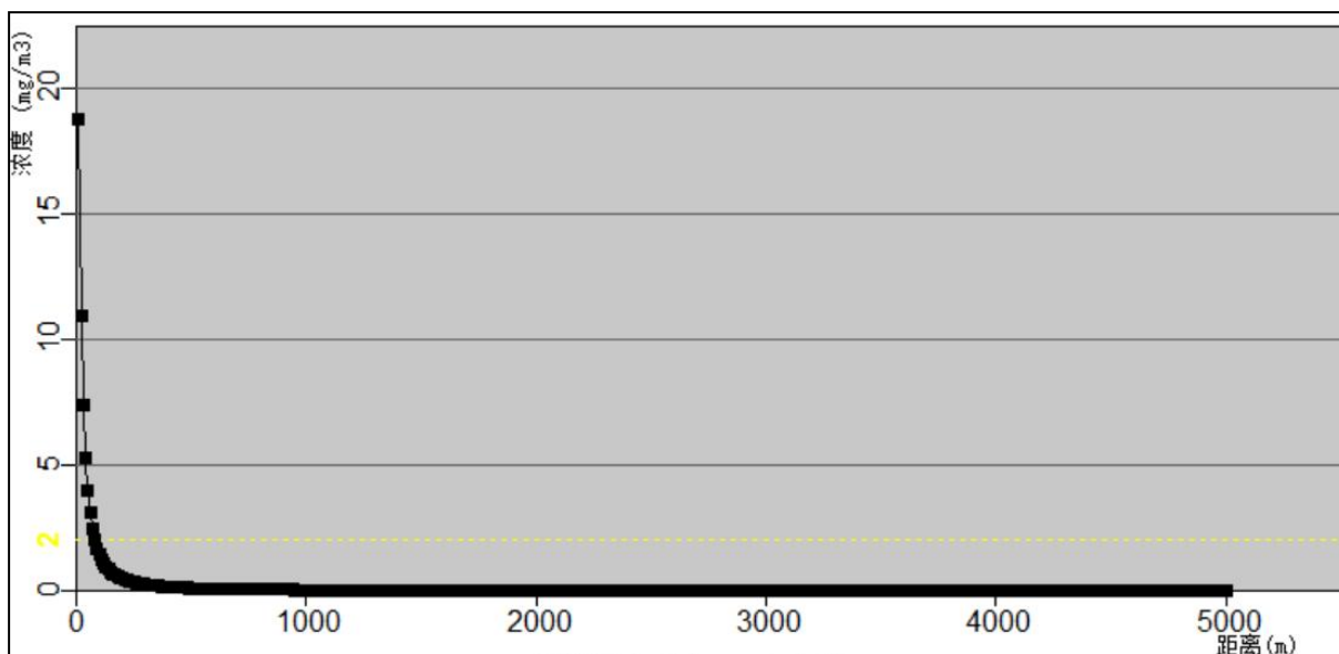
图 6.1-1 二氧化硫浓度随距离的变化曲线图
