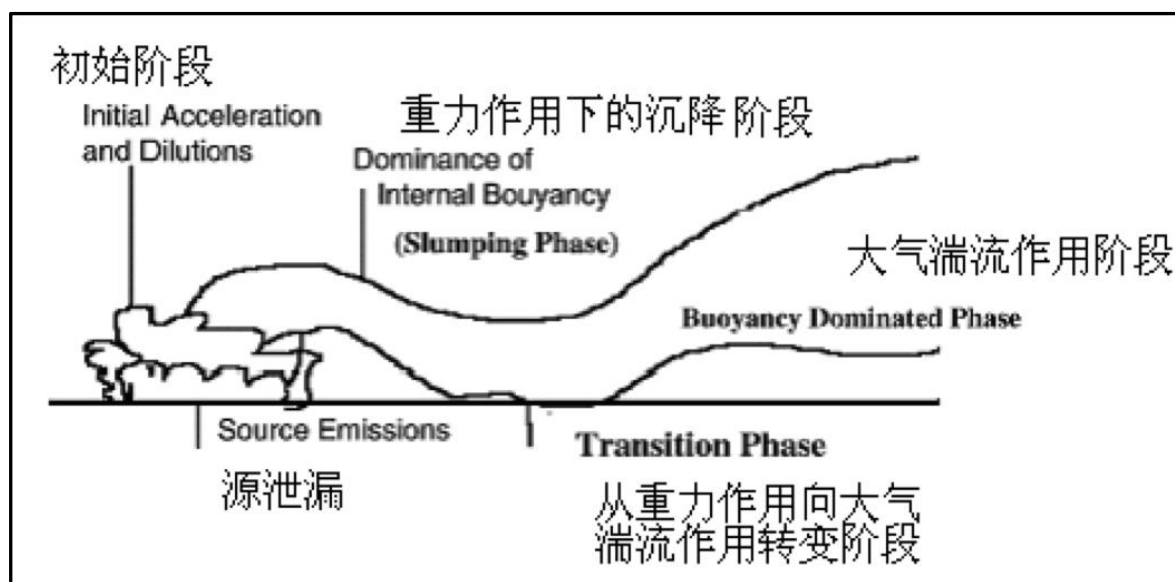
图 5.2-1 泄漏事件大气扩散过程
