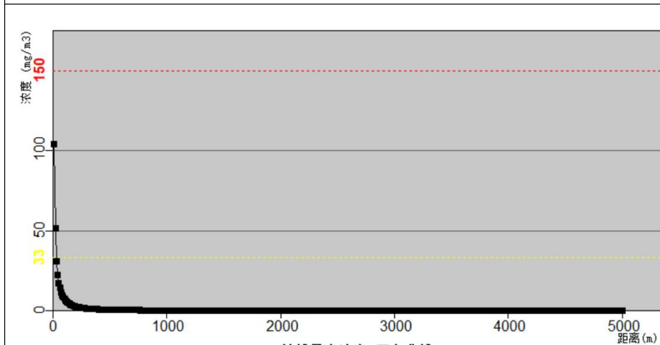
图 6.1-5 氰化氢浓度随距离的变化曲线图
