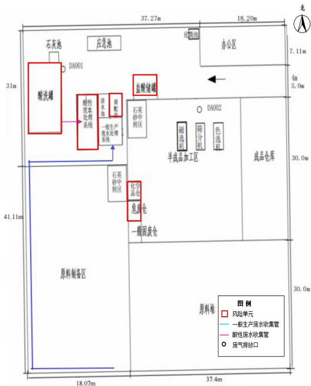
图 4.4-1 厂区内危险单元分布图
