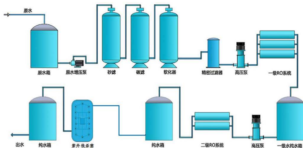
图 2-4 纯水制备工艺流程图
