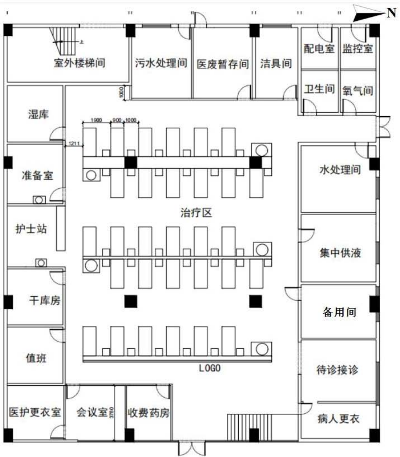
附图 5 项目平面布局图
