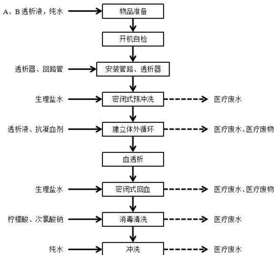
图 2-3 血液透析治疗工艺流程图及产排污环节图
