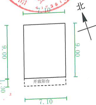
罗定市连州镇云致村委南山53号 欧炉南建房平面图
