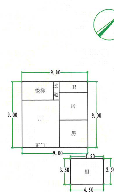
注:1、首层占地面积:96.75m 2 2、总建筑面积:278.11m 2
