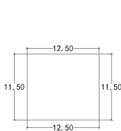
首层平面图 1:200
